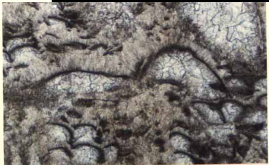
照片 III-1-【8】 层纤结构 图为珊瑚鳞板，它由隐粒层（黑色）和垂直向上生长纤体构成的层纤结构组成。内腔为亮晶方解石充填。 塔西南P1 单偏光 照片长边长2 mm
